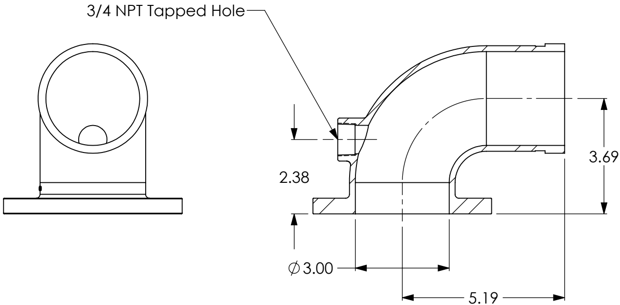
SECTION A-A
