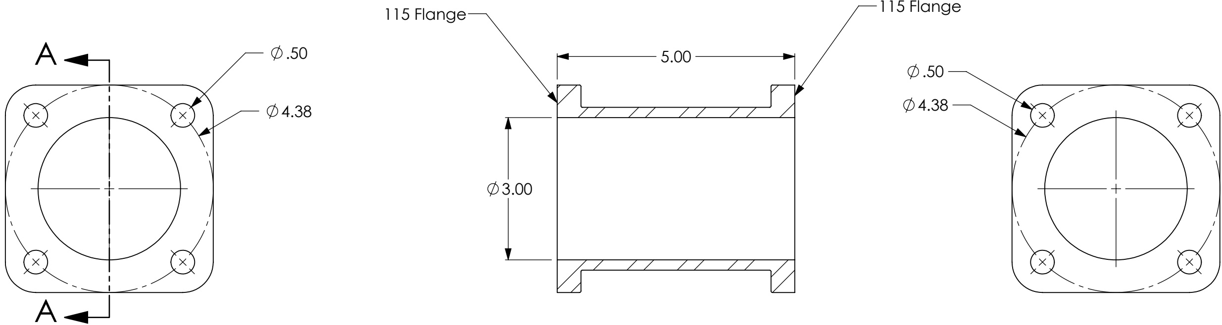
SECTION A-A
