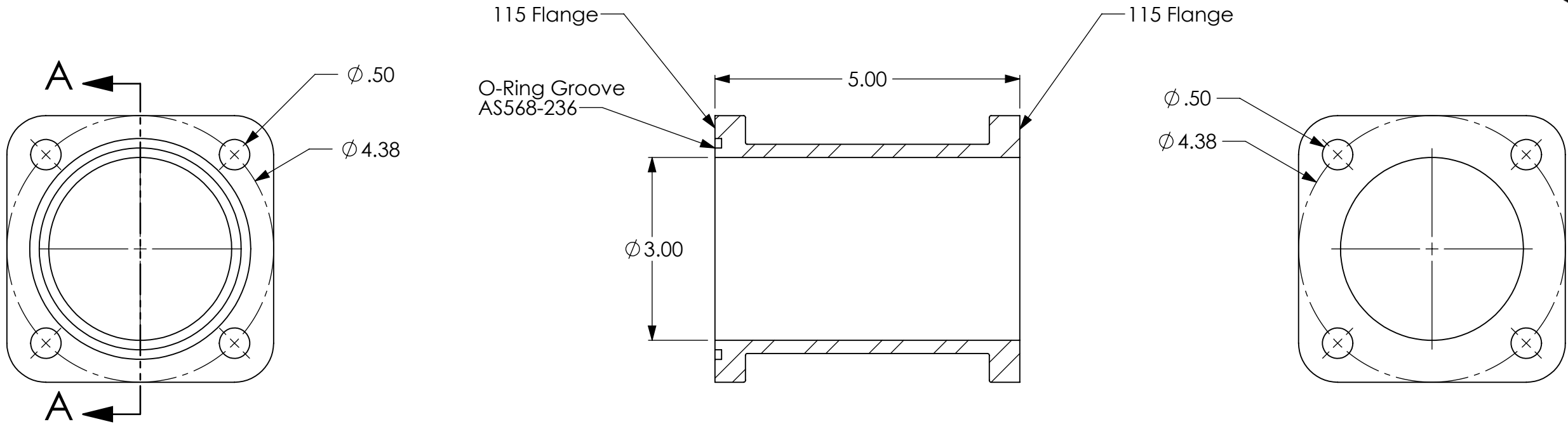
SECTION A-A
